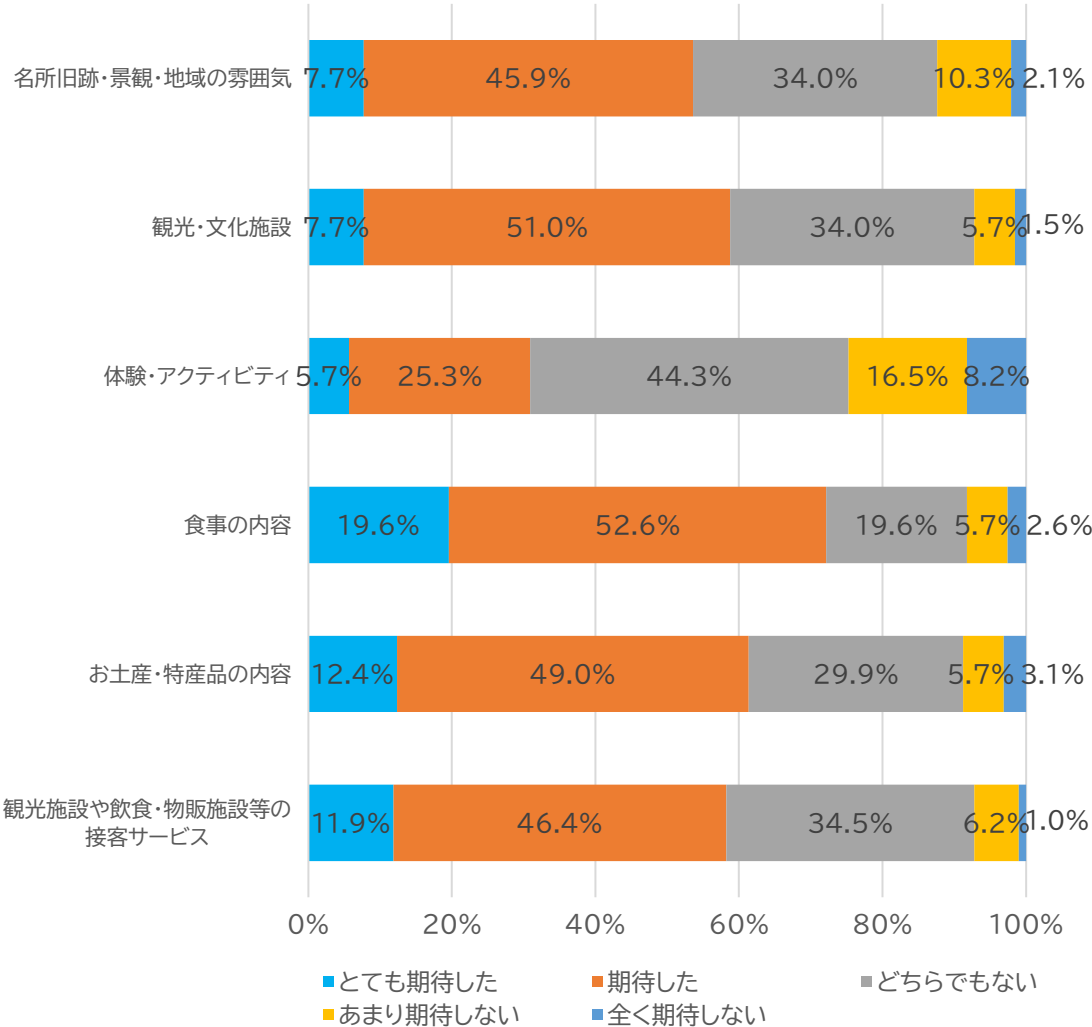
期待度
