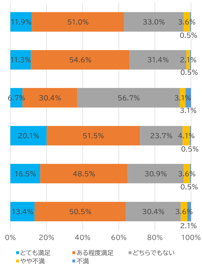
満足度
